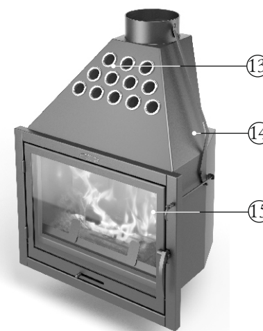
Рисунок 2. Общий вид и расположение основных элементов каминной топki «Аквариус».
