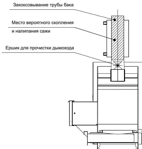
Рис.5 Схема прочистки печи
