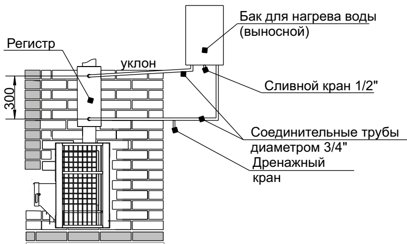
Рис.2 Печь «БУГРИНКА» с дистанционным нагревом воды
