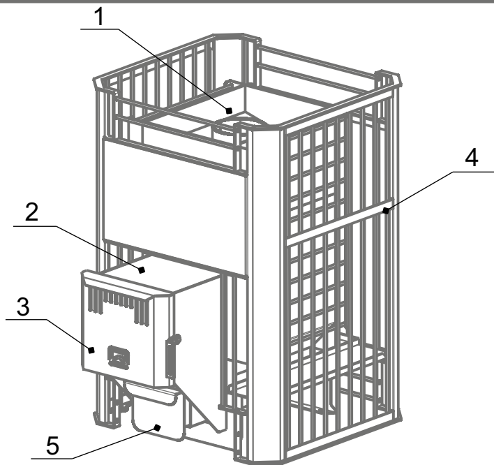
Рис.1 Конструкция печи «БУГРИНКА»
