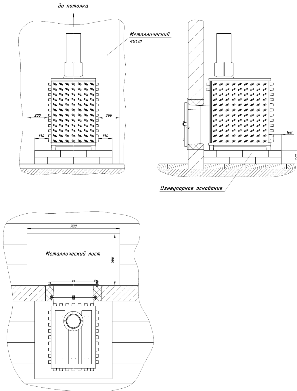
Рис.3 – Монтаж печи
