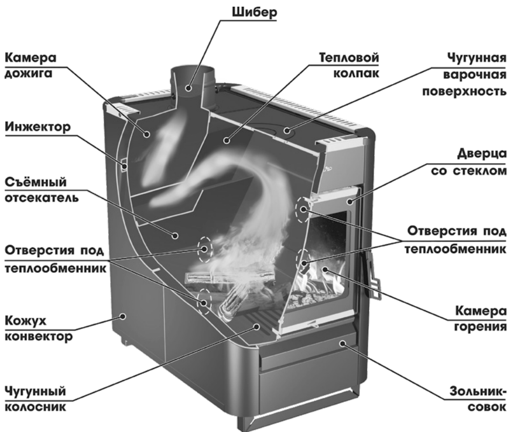
Рисунок - 1. Устройство печи-камина «Садовый» ОВ/ЧП/С (Т).
