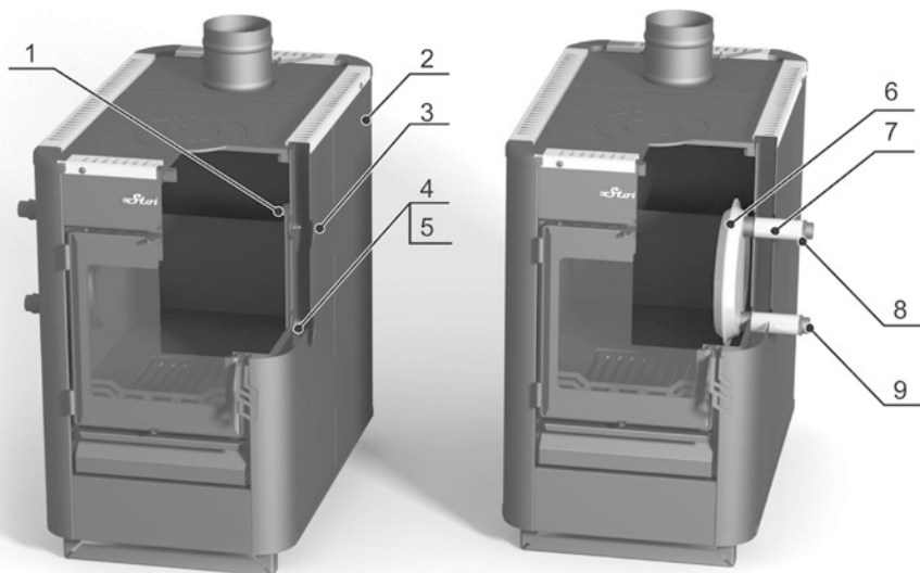
Рисунок-3. Установка теплообменника.
