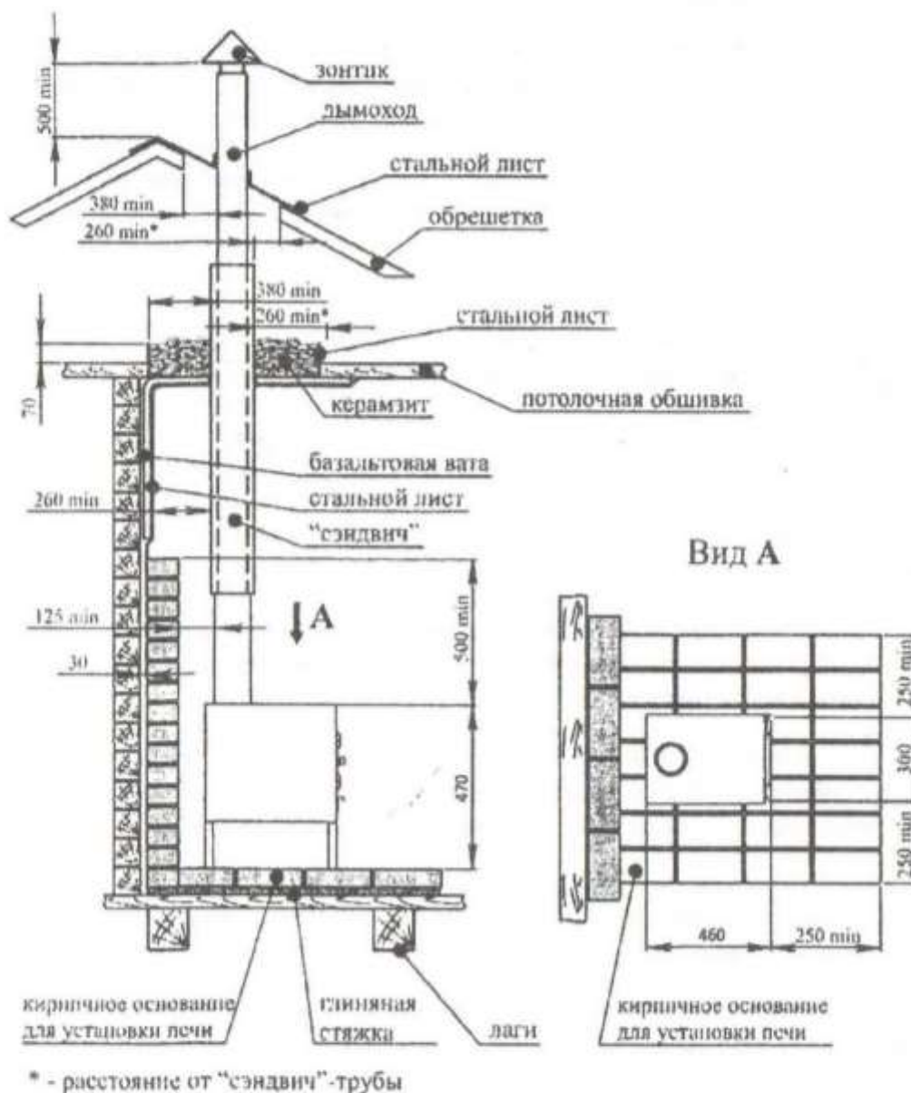
Рис. Схема установки печи
